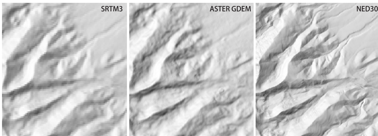
中央コロラドの山岳地帯の起伏陰影画像。シャトルレーダ地形図ミッションのバージョン 3 の DEM データ (SRTM3、セルサイズ 3 秒、左)、ASTER GDEM (セルサイズ 1 秒、中央)、および米国のナショナル標高データセット (NED30、セルサイズ 1 秒、右) の比較。ASTER GDEM と NED30 の画像は 1 倍ズームで表示されています。ASTER GDEM のセルサイズは約 30m ですが、右上の扇状地にある細い水路のような 100 ~ 120m より小さな地形は ASTER GDEM でははっきり見えません。ASTER GDEM の実効的な空間解像度はセルサイズ 90m の SRTM3 DEM と同程度です。
